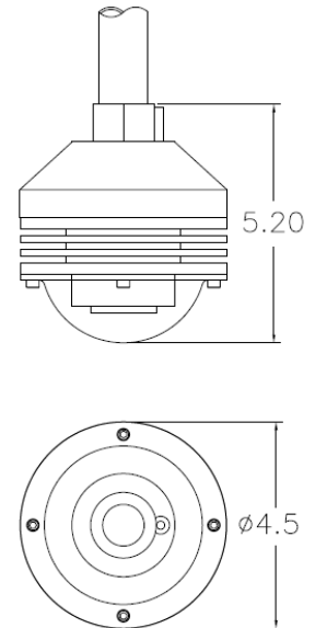
Pendant Mount
